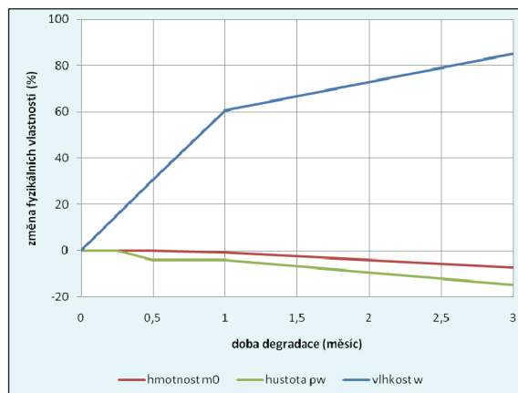
8: Grafické znázornění procentuální změny fyzikálních vlastností v závislosti na čase u Serpula lacrymans
